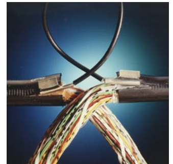
Jonction de blindage souple
