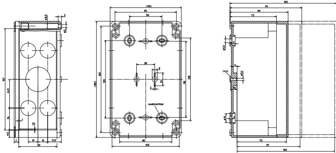
Katalogzeichnung: TK 1811
