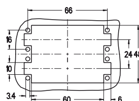
Montageausschnitt
