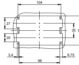
Montageausschnitt
