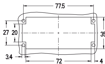
Montageausschnitt
