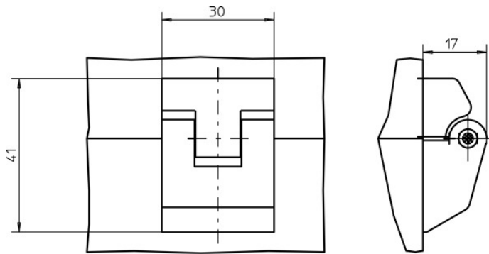
Aussenscharnier AL-Serie Art.-Nr. 154 210 01
