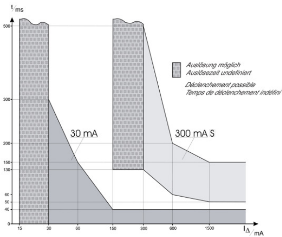
Abschaltzeiten eines unverzögert und eines verzögert (selektiv) ansprechenden RCCBs der Baureihe DFS 4
